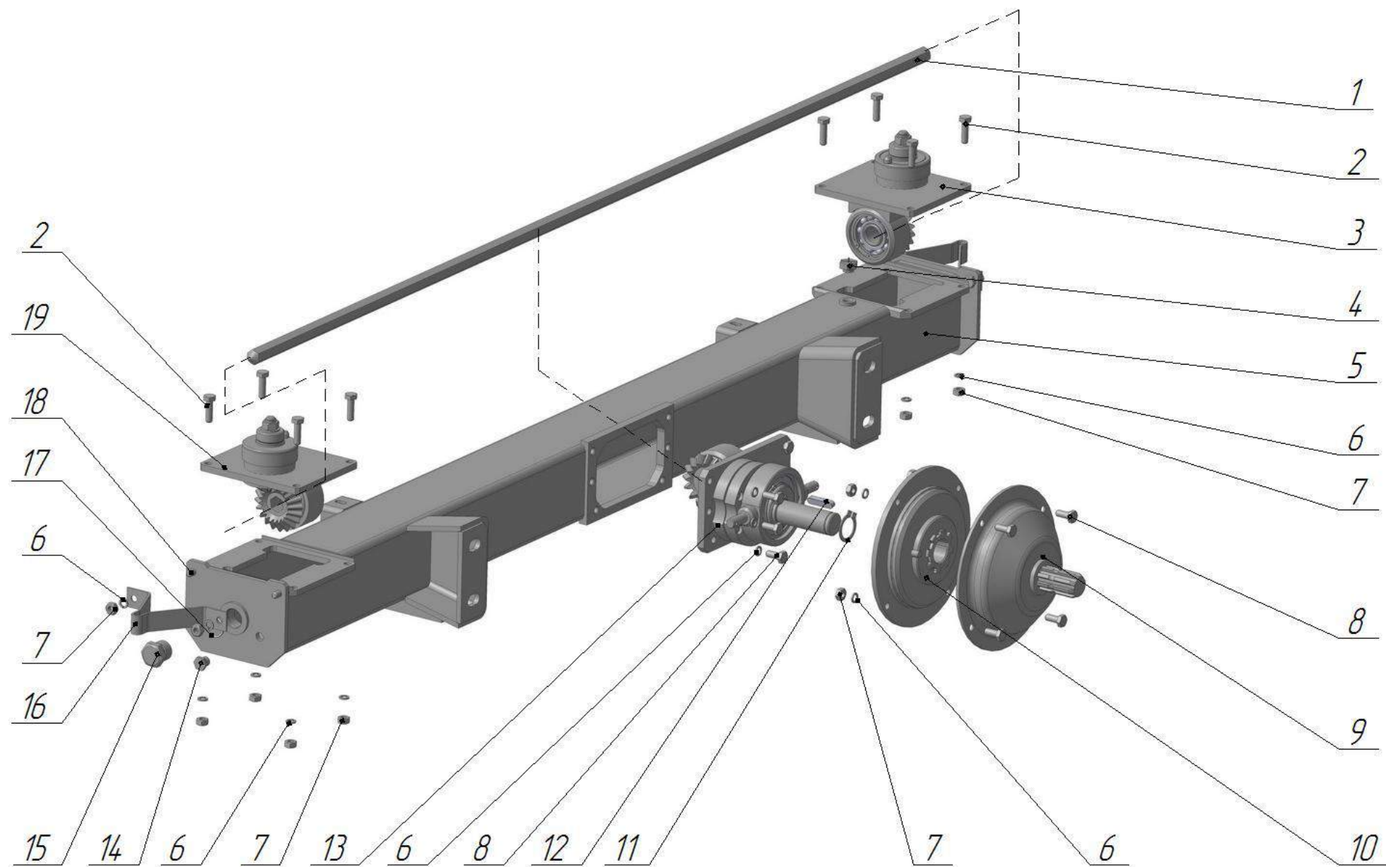
Рисунок 9 – Привод
