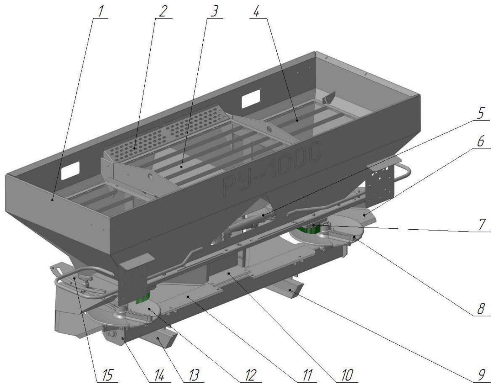
Рисунок 1 – Рассеиватель удобрений минеральных РУ-1000 agro-parts.org
