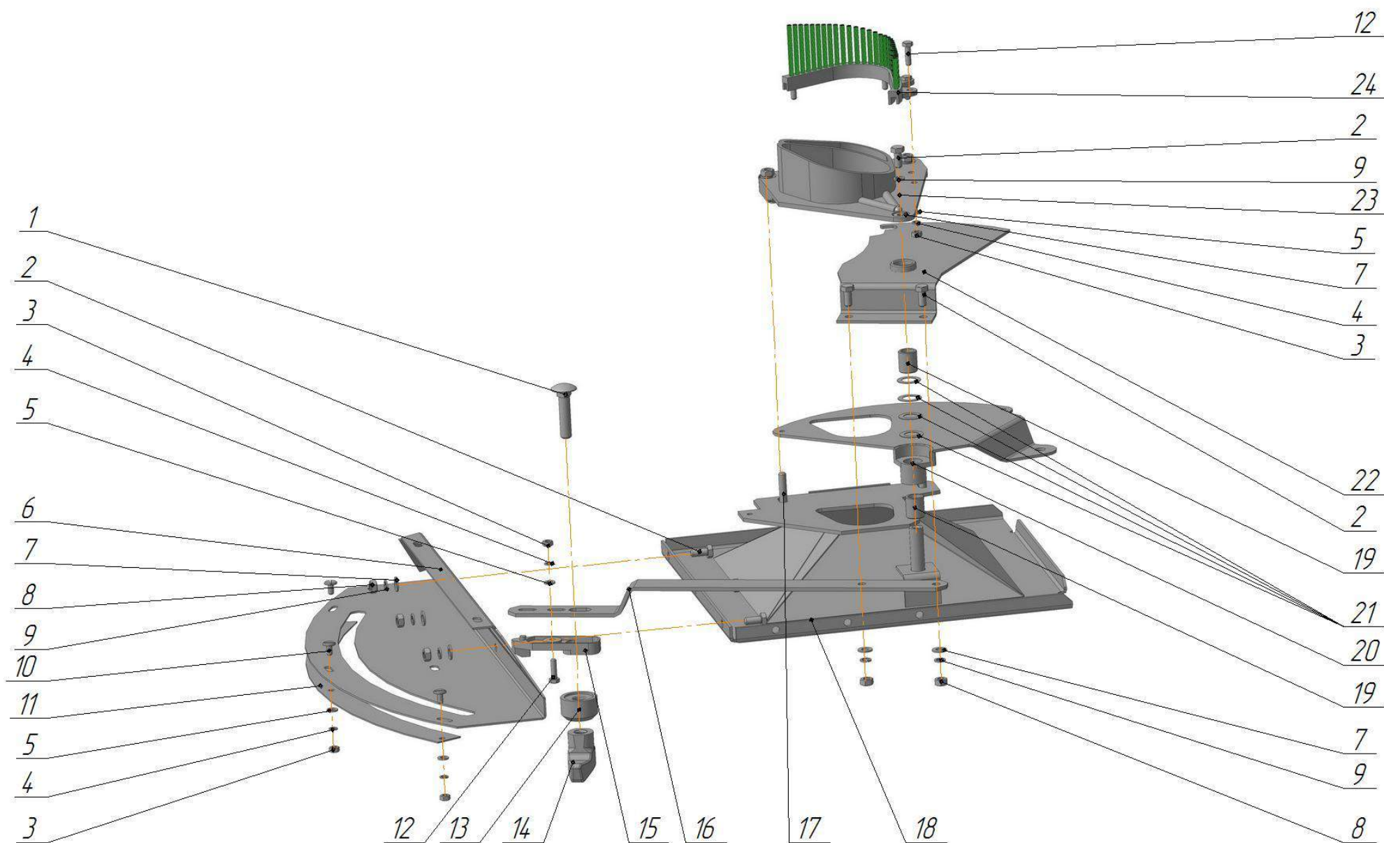
Рисунок 7 – Узел дозирующий agro-parts.org
