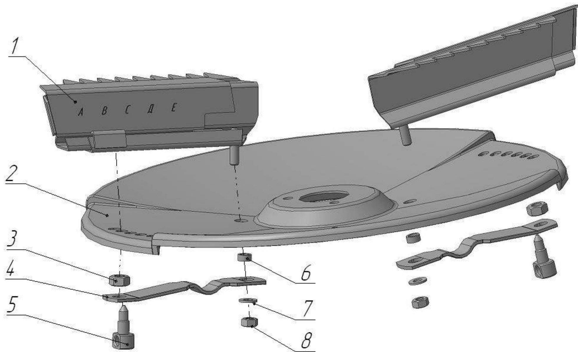
Рисунок 5 – Метатель
