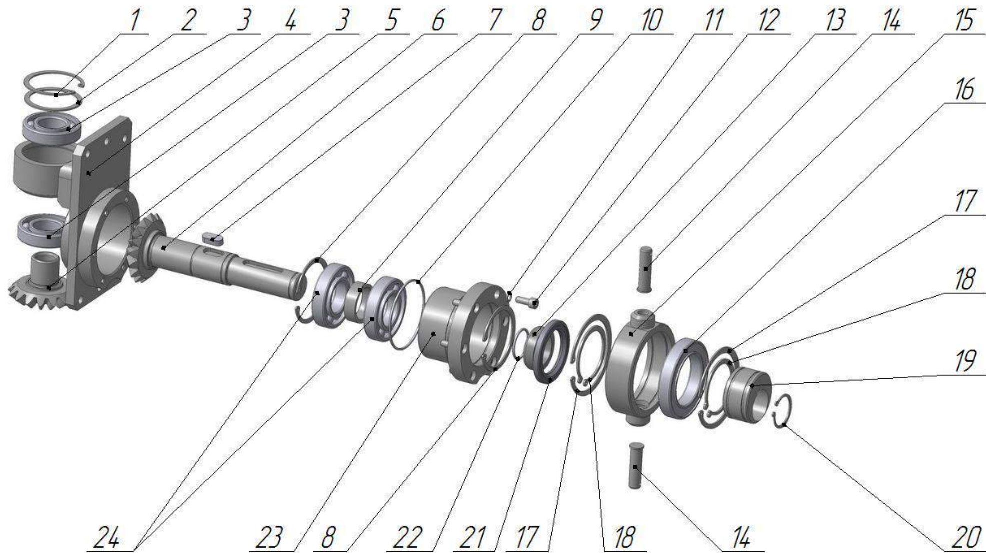
Рисунок 11 – Передача коническая
