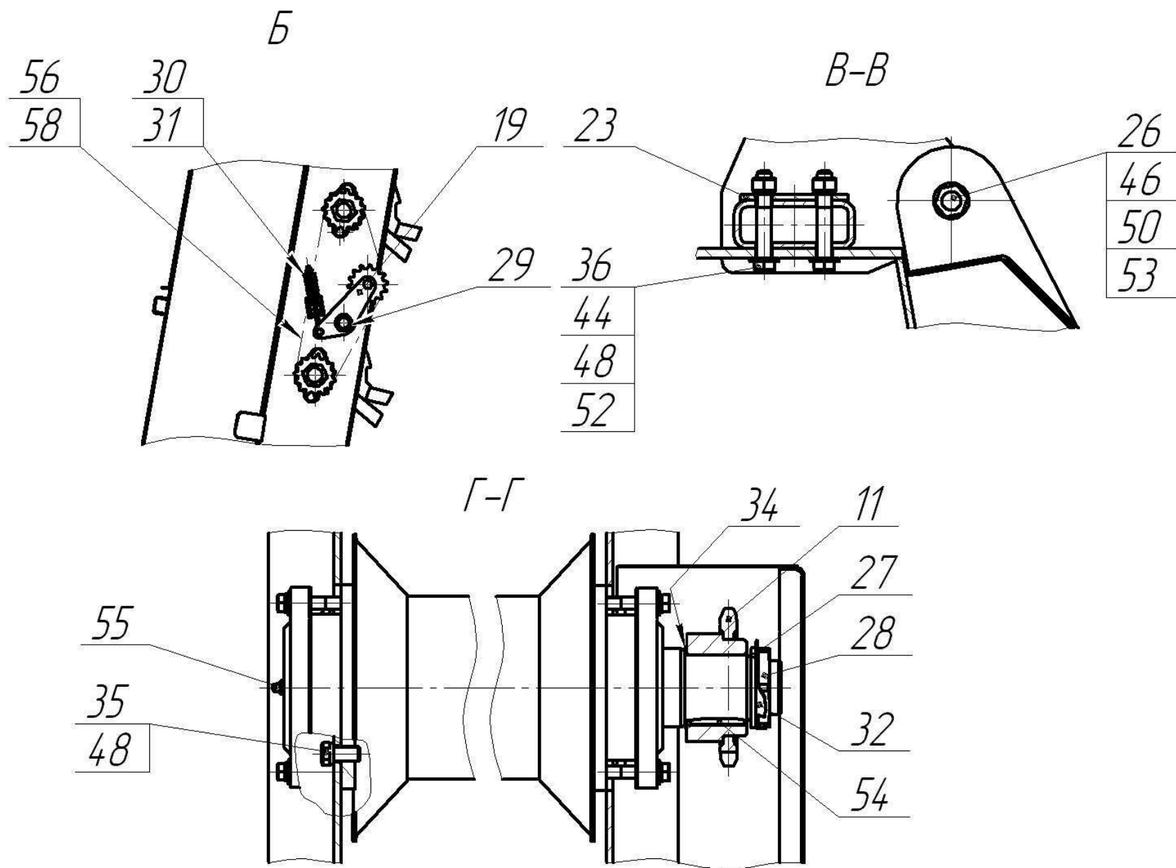
Рисунок 6.1 – Разбрасыватель (МТУ-15.07.00.000)
