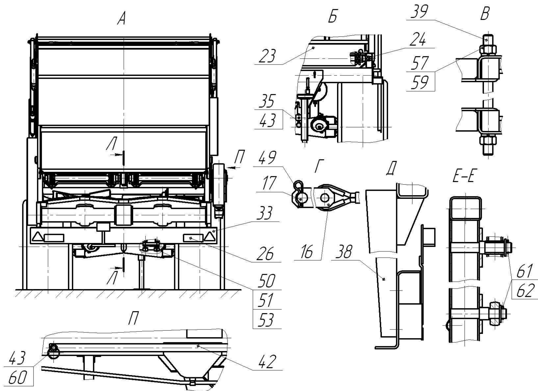
Рисунок 2 – Машины МТУ
