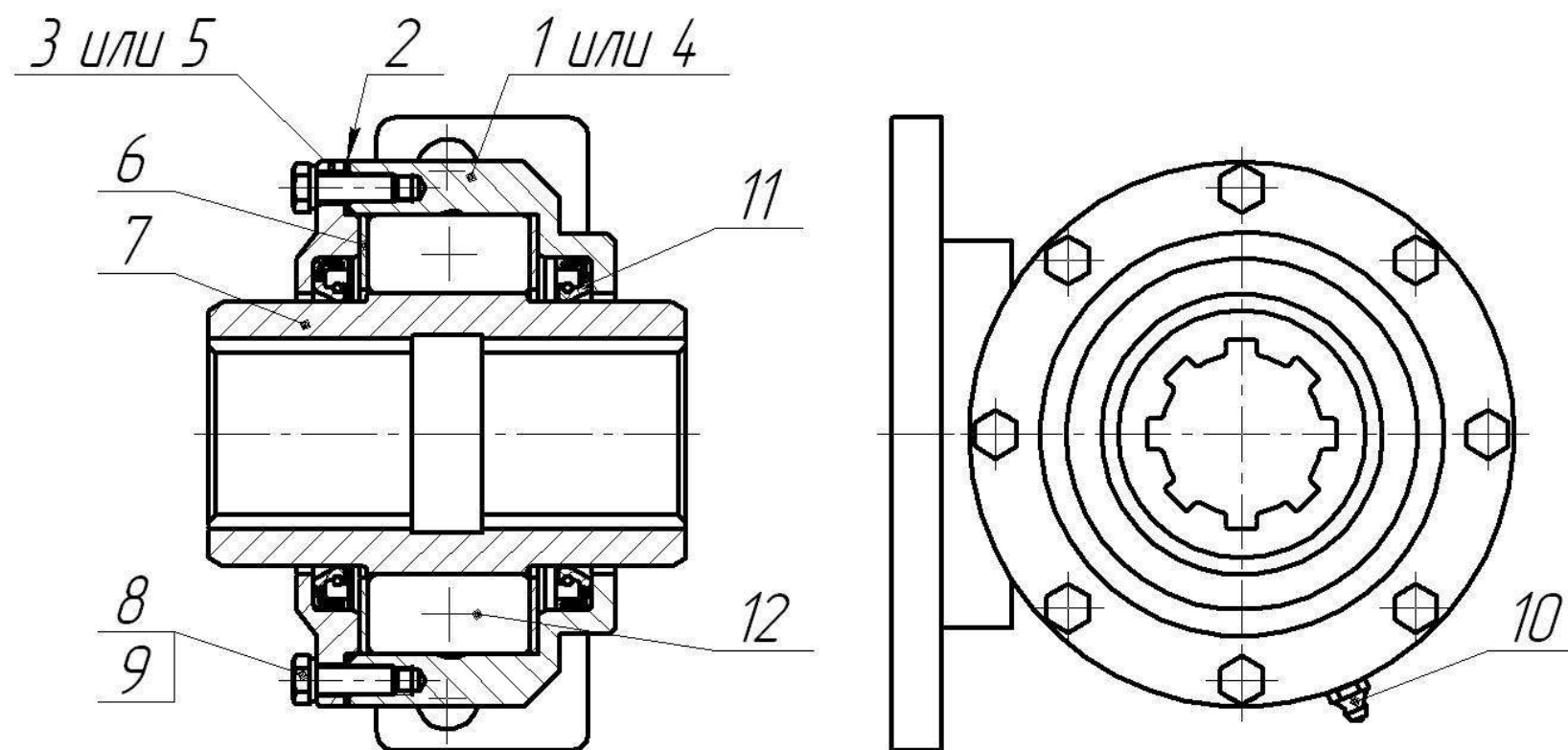
Рисунок 11.6 – Опора (ПС-60.05.03.000-01)
