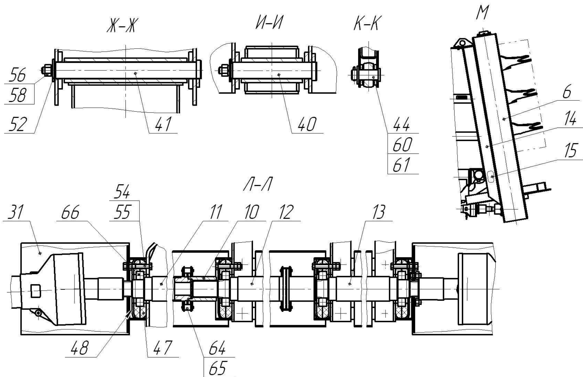
Рисунок 3 – Машины МТУ
