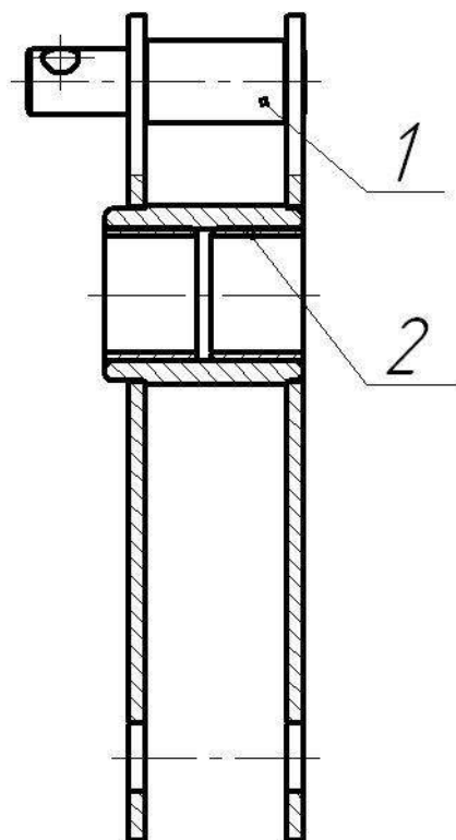
Рисунок 6.8 – Кронштейн (ПРТ-7А.07.09.040)
