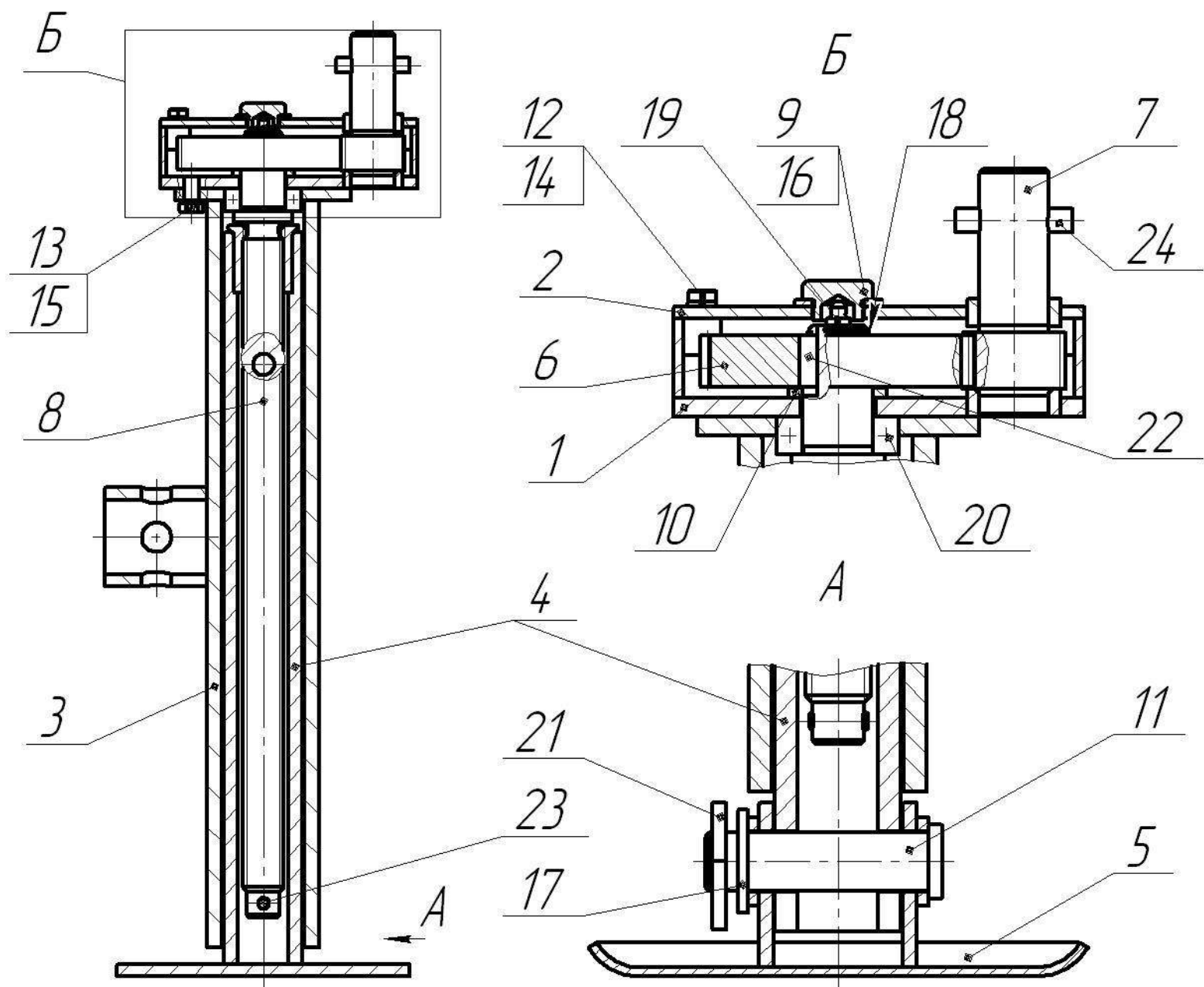
Рисунок 5 – Опора регулируемая (MTU-15.05.00.000 / MTU-15.05.00.000-01)
