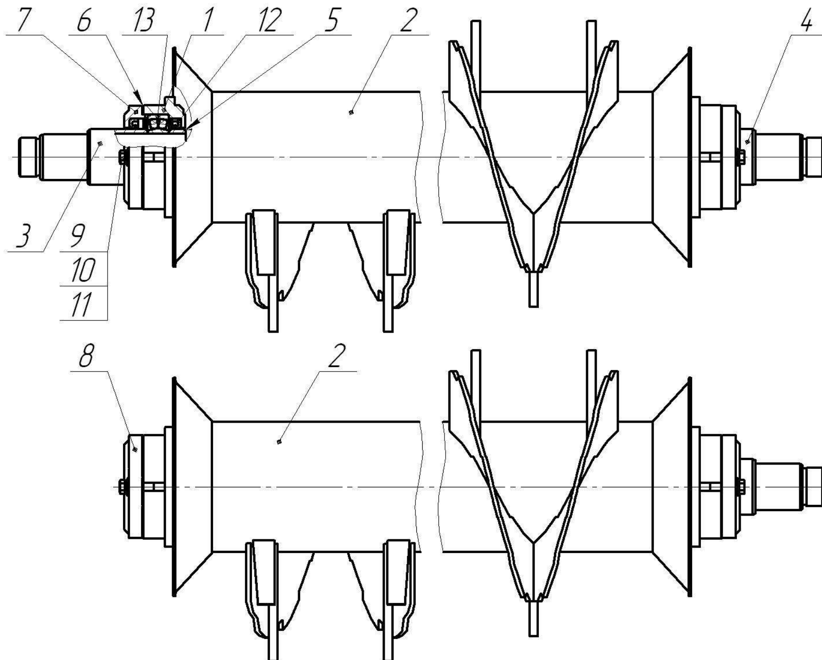
Рисунок 6.6 – Шнек (МТУ-13.02.32.000 / МТУ-13.02.32.000-01)
