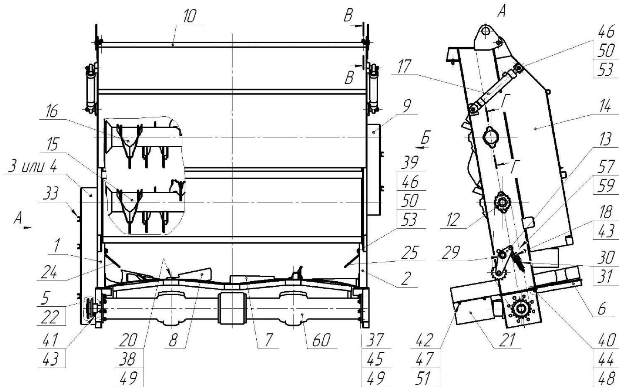
Рисунок 6 – Разбрасыватель (МТУ-15.07.00.000)
