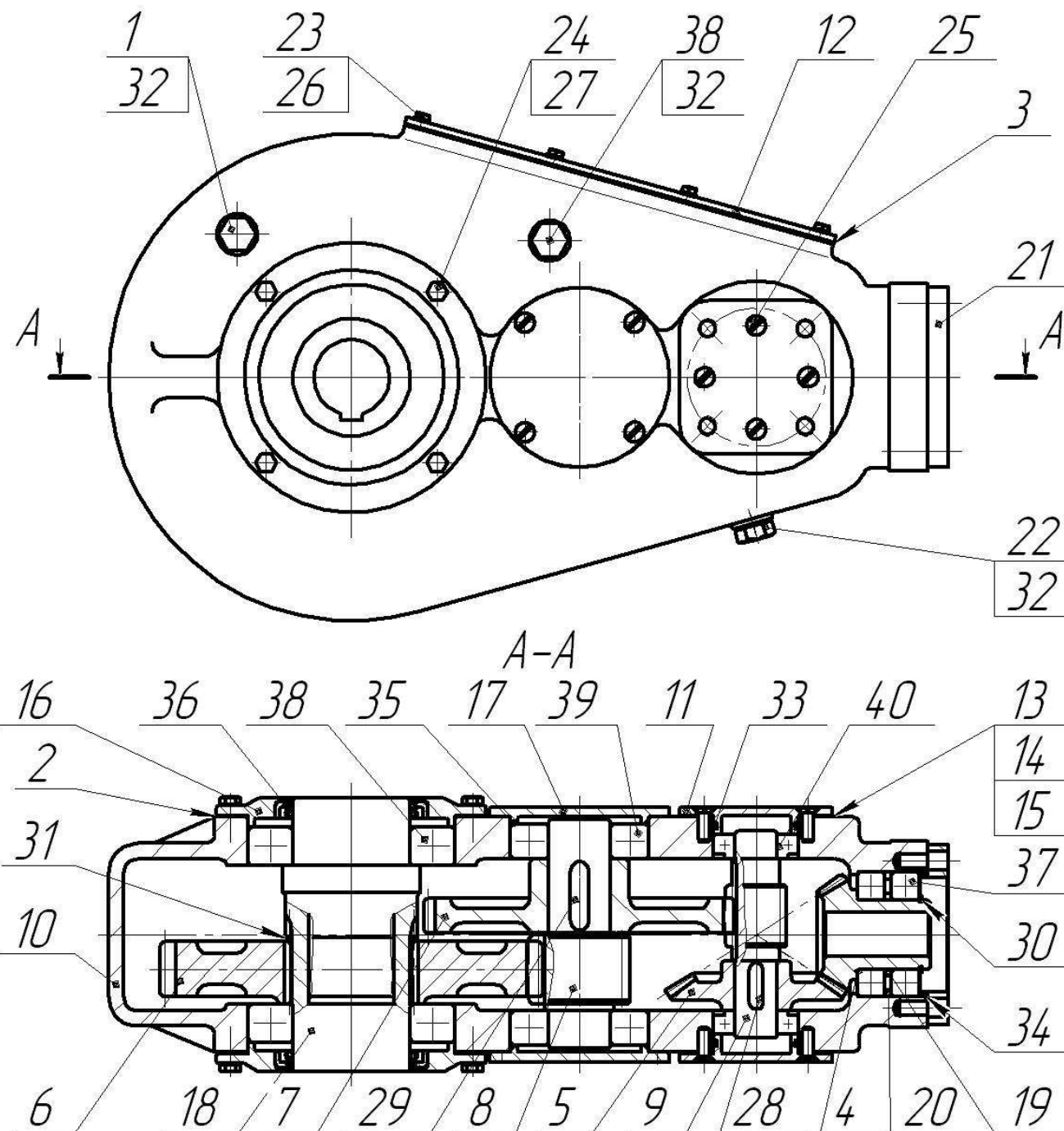
Рисунок 11.4 – Редуктор (MTU-13.16.05.000)
