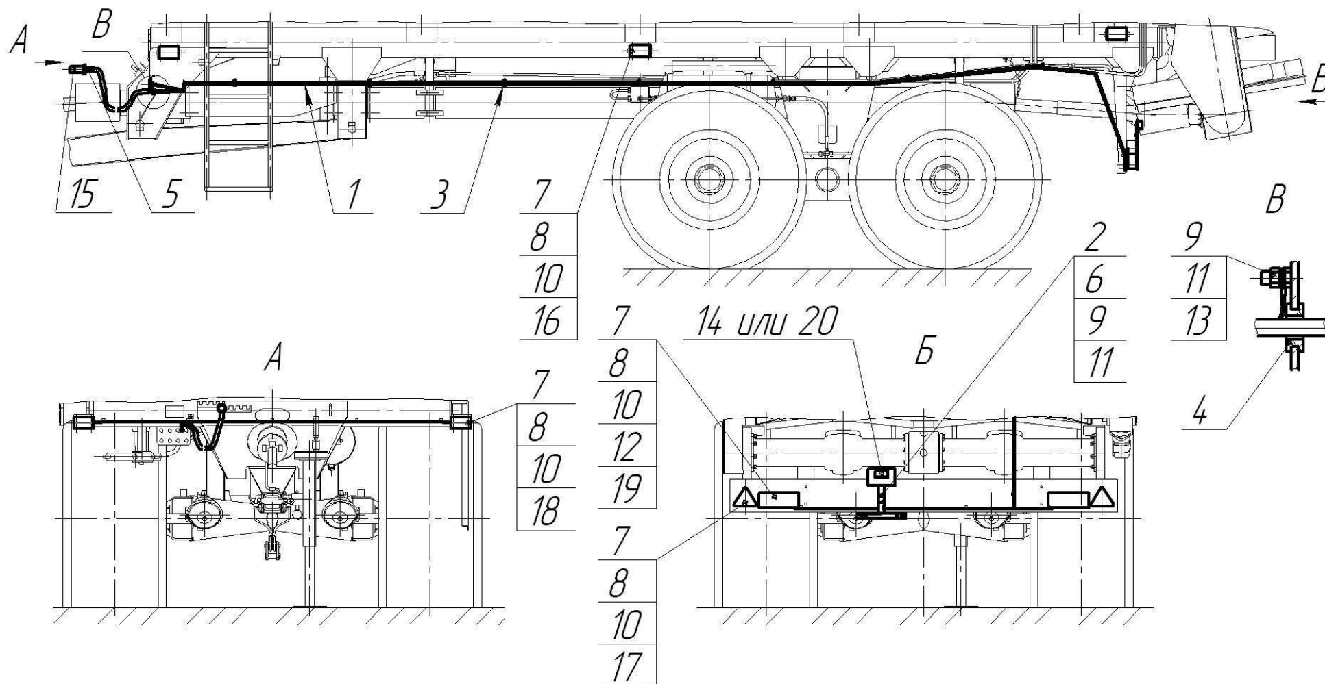
Рисунок 13 – Электрооборудование (MTU-13.19.00.000)
