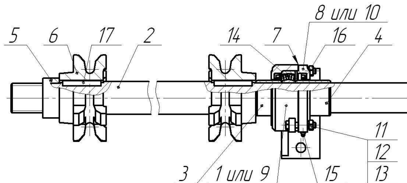
Рисунок 11.2 – Вал ведущий (МТУ-13.16.02.000)
