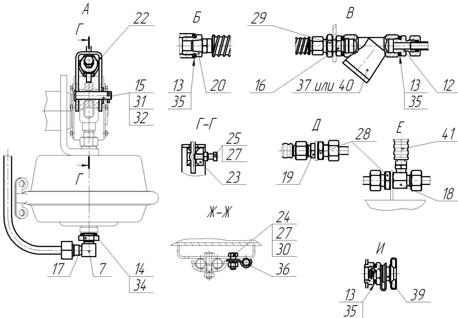
Рисунок 12.1 – Система тормозная (МТУ-13.18.00.000)
