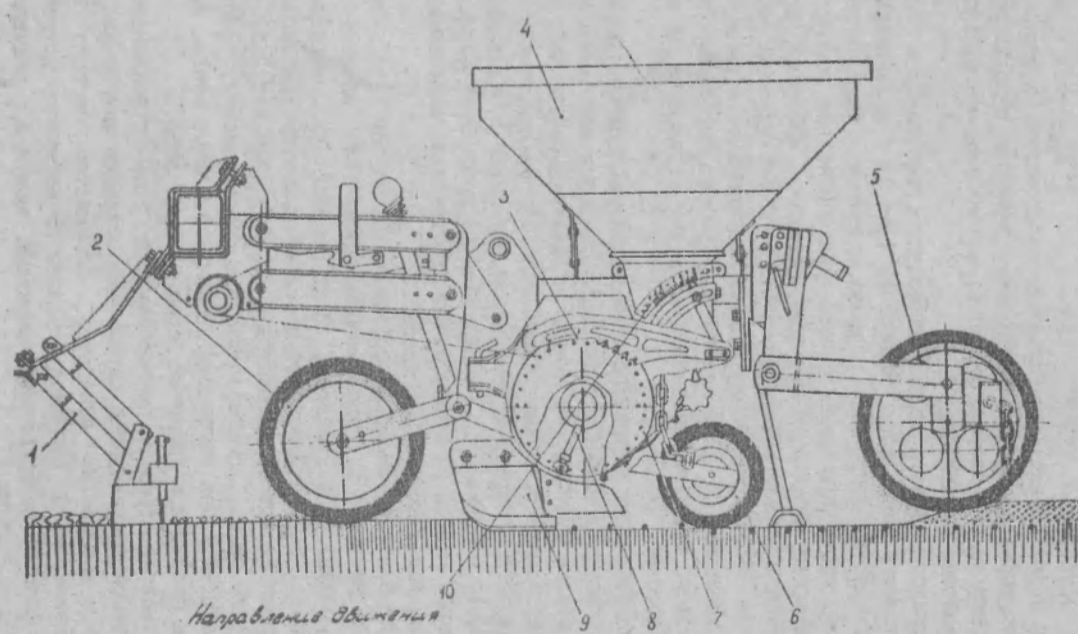
РИС. 4. ТЕХНОЛОГИЧЕСКАЯ СХЕМА РАБОТЫ СЕВКИ 1 - КОМБИНИРОВАН; 2 - ПЕРЕДНЕЕ СЛОНОВОЕ КОЛЕСО; 3 - СЕПАРАТОР; 4 - БУНКЕР ДЛЯ СЕМЕНИ; 5 - ЗАДЕЛЫВАЮЩЕЕ КОЛЕСО; 6 - ПРИКАТЫВАЮЩЕЕ КОЛЕСО; 7 - ВЫЖИВАЮ- ЩИЙ ДИСК; 8 - РОТЛИК; 9 - СКОБЛИК; 10 - ШКАЛА РЕГУЛИРОВКИ СЕПАРАТОРА
