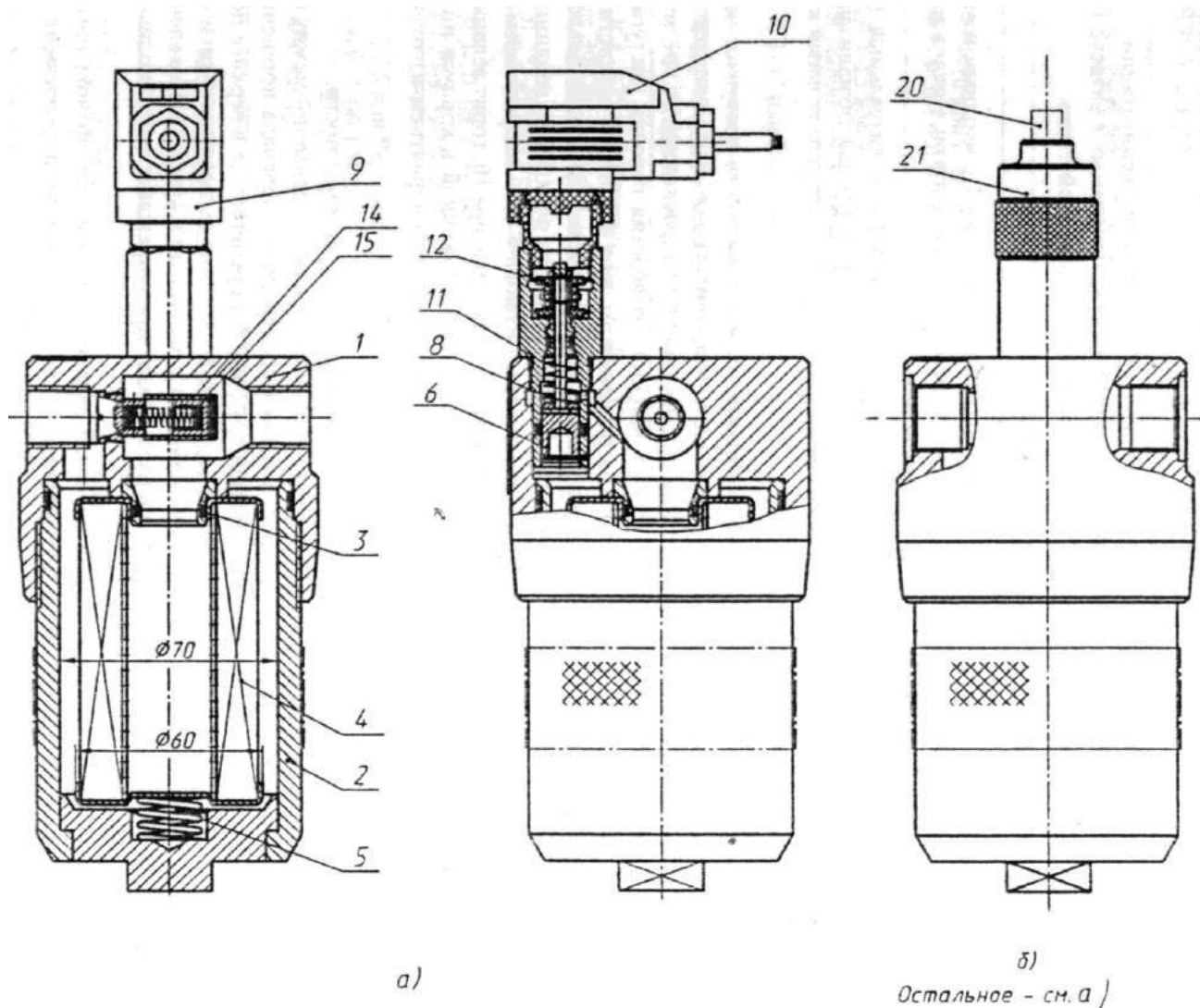
Рисунок Л.2 – Фильтр напорный ФГИ20/3-10КВ (МВ)
