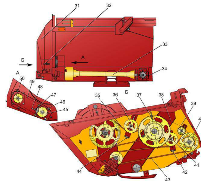
Приводы жатки
