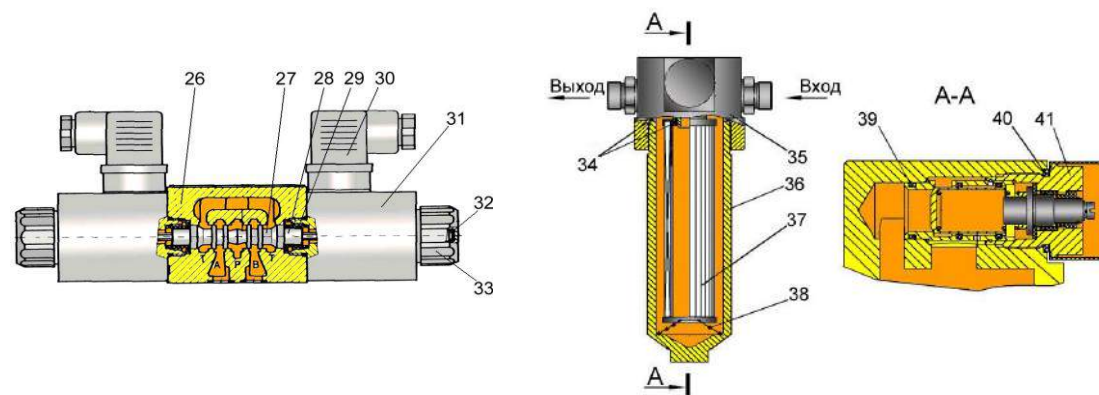
Гидрораспределитель
