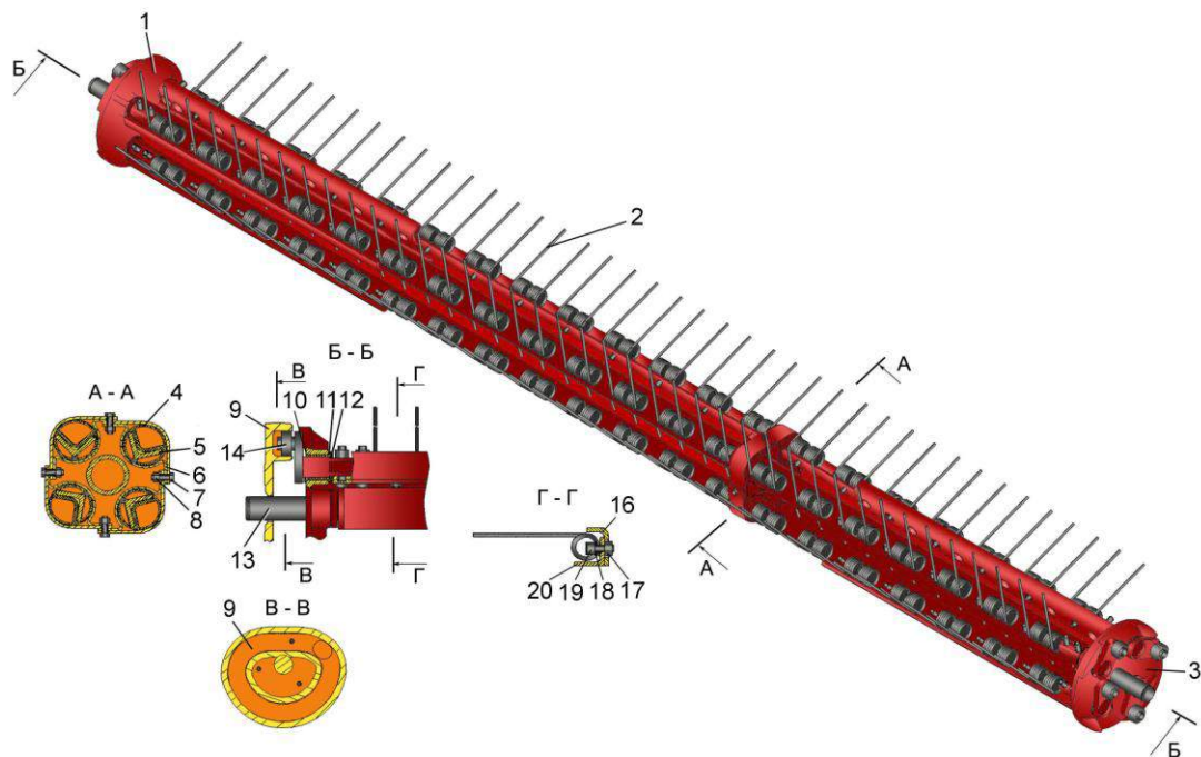
Устройство подбирающее
