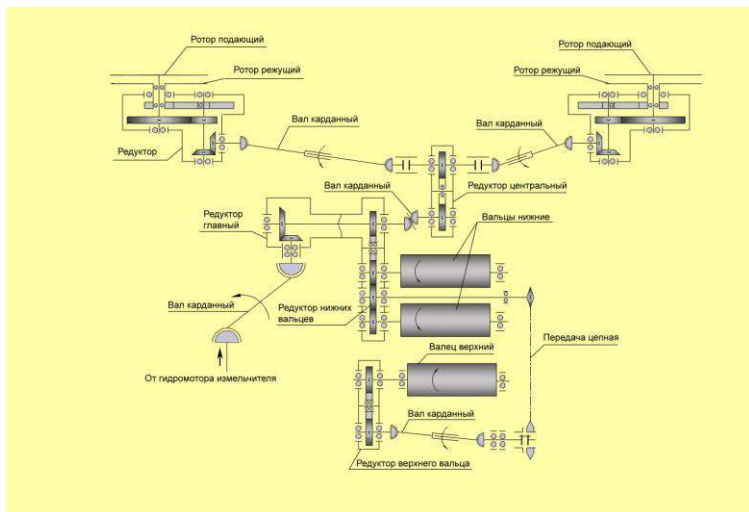
Схема кинематическая принципиальная жатки для грубостебельных культур
