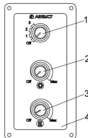
Рисунок 1.38 – Панели кабины
