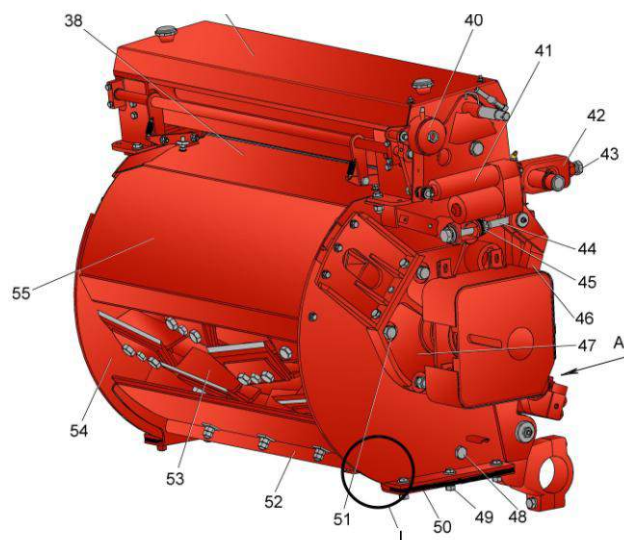
Измельчающий аппарат
