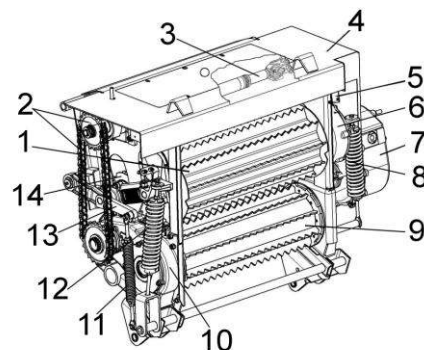
Рисунок 1.21 - Питающе-измельчающий аппарат
