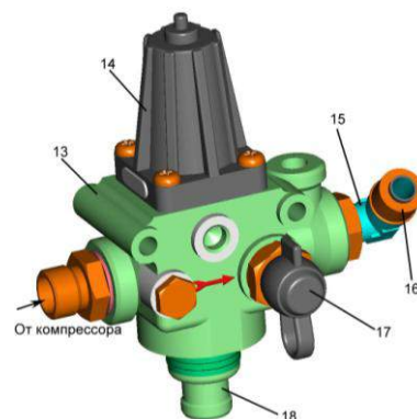
Регулятор давления
