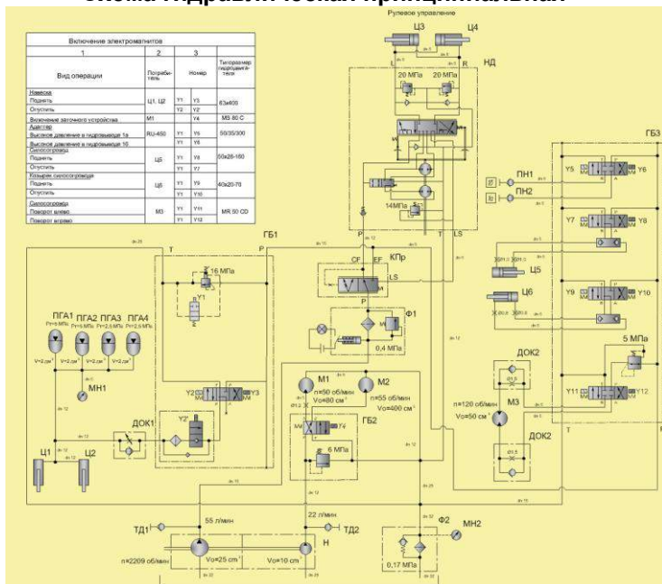
Схема гидравлическая принципиальная
