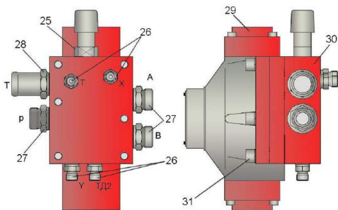
Гидроблок адаптеров
