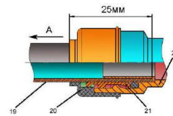
Фитинг
