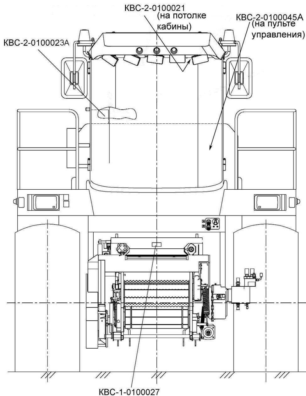
Знаки безопасности на измельчителе самоходном (вид спереди)
