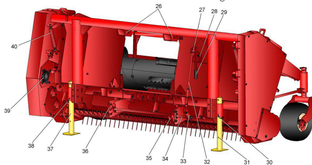
Навеска подборщика
