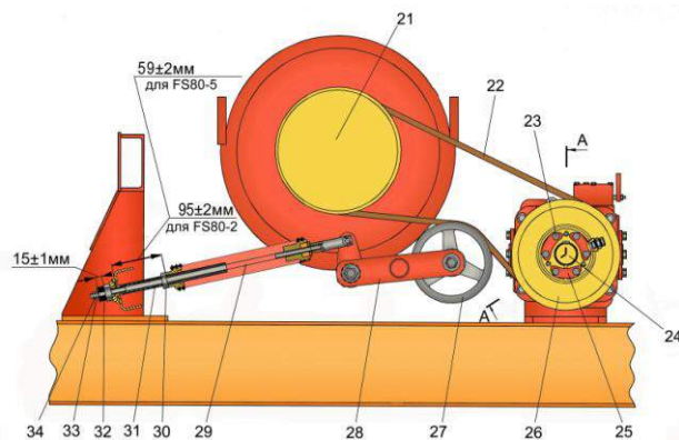
Привод гидростата
