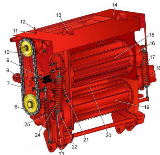
Питающий аппарат
