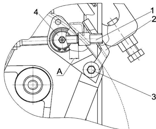
Рисунок 2.7 – Отвод питающего аппарата от измельчающего
