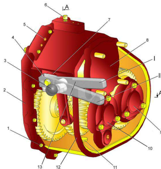
Коробка передач
