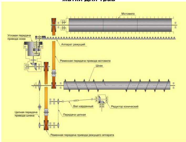
Схема кинематическая принципиальная жатки для трав
