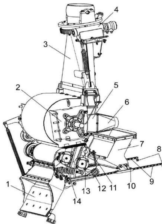
1 – камера приемная; 2 – ускоритель выброса; 3 – основание силосопровода; 4 – механизм поворота силосопровода; 5 – воздуховод; 6 – переходник; 7 – проставка; 8, 10, 11 – болты; 9 – цепь; 12 – механизм перемещения; 13 – скоба; 14 – устройство доизмельчающее
