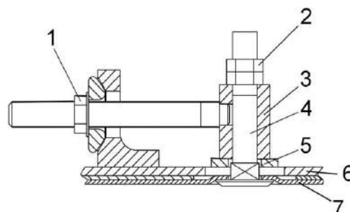
1, 2 – гайки; 3 – стяжка; 4 – болт; 5 – шайба; 6 – трубопровод; 7 – вставка
