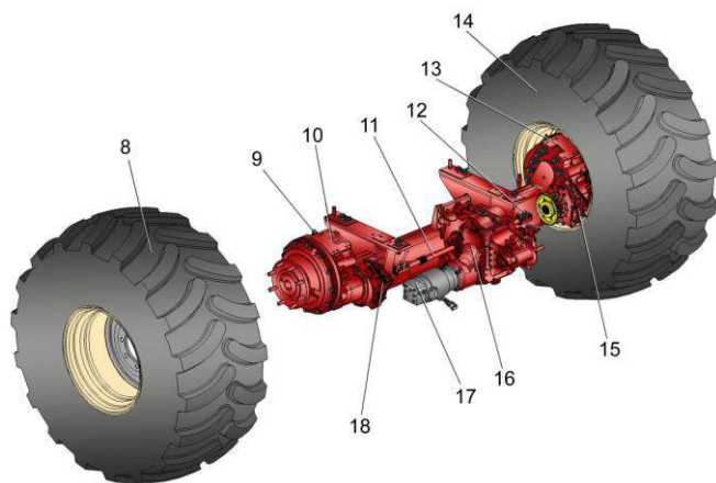
Мост ведущих колес
