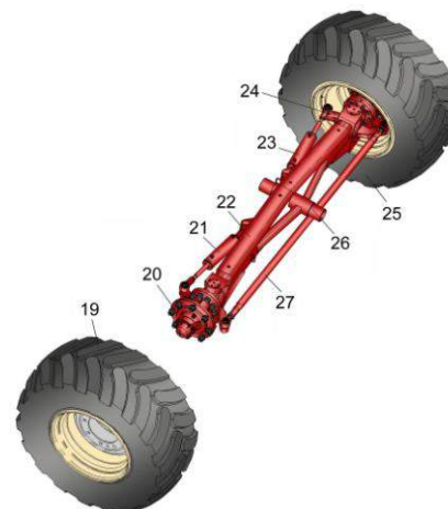
Мост управляемых колес
