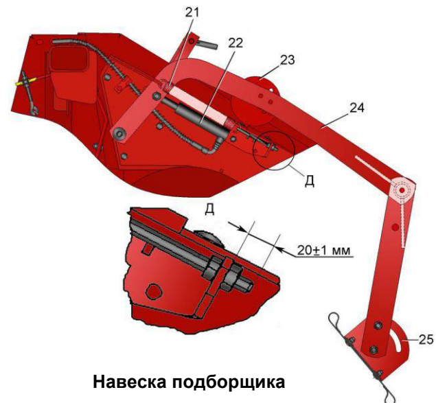
Прижимное устройство
