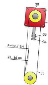
Навеска жатки на самоходный измельчитель
