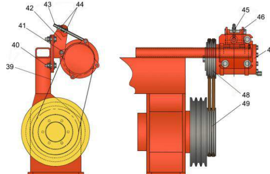
Привод компрессора
