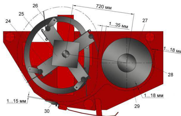
Регулировка положения шнека и мотовила
