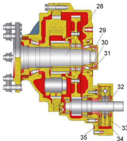
Бортовой редуктор
