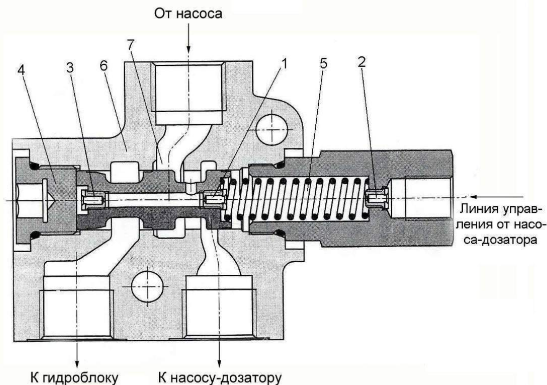
Рисунок 1.31 – Приоритетный клапан
