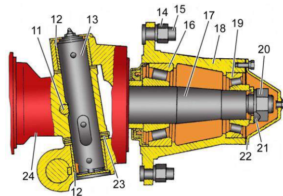
Поворотный кулак
